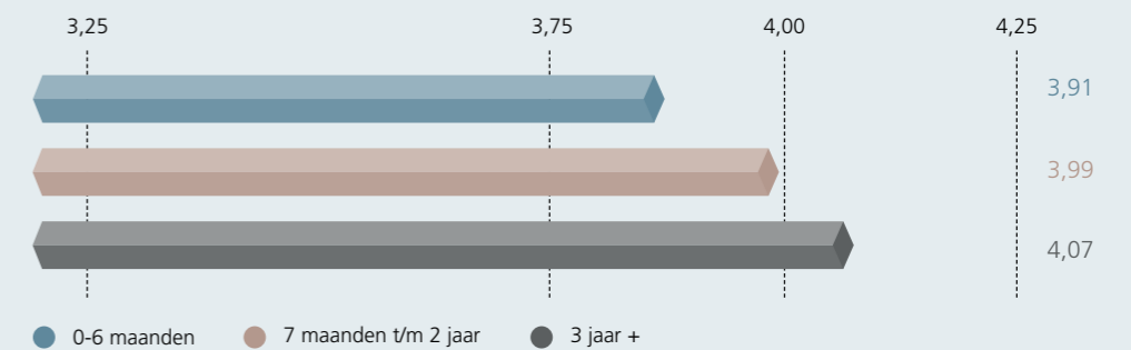
Figuur 2 Relationele vaardigheden: Verschil scores gemiddeld over de tijd op relationele vaardigheden.
